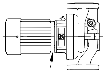
Fig. 25 Drain hole
